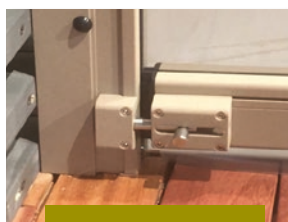
PARTICOLARE CATENACCIO
